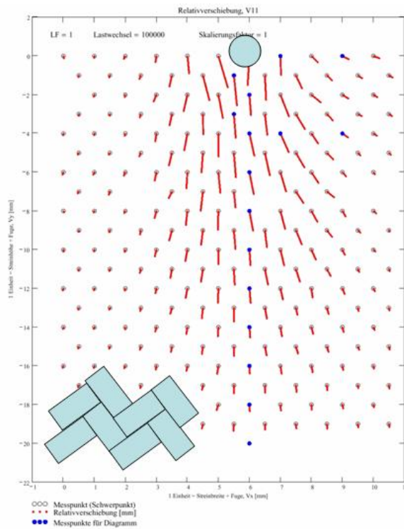
Rechtecksteine, Fischgrätverband (gute Lastverteilung)
