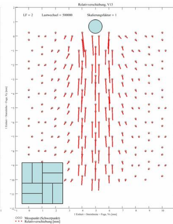
Rechtecksteine, Parkettverband (schlechte Lastverteilung)
